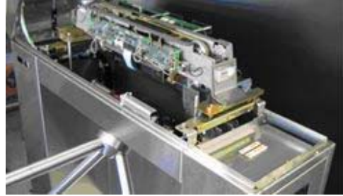
Validador de bilhetes magnéticos da T'Trans
